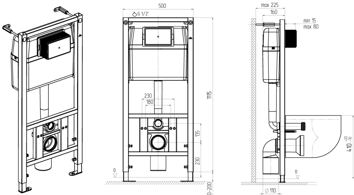
рис.1 Габаритные размеры и параметры установки скрытой установочной системы подвесного унитаза
